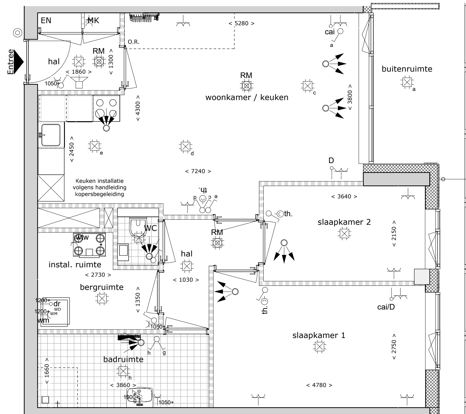
Bouwnummer A012 1 : 50
