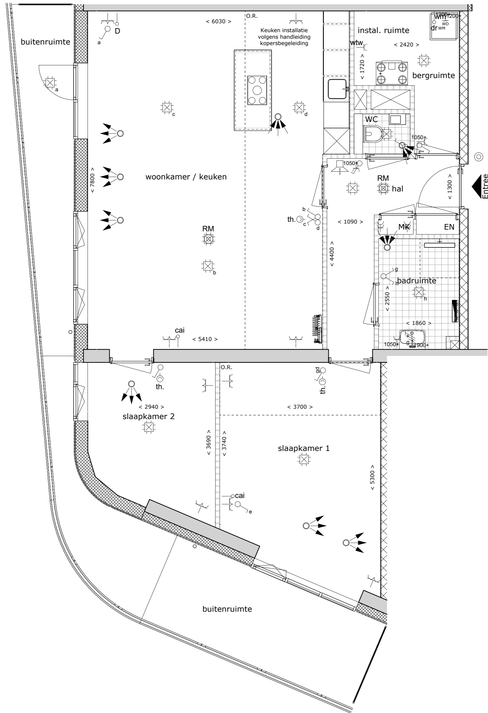
Bouwnummer A016 1 : 50
