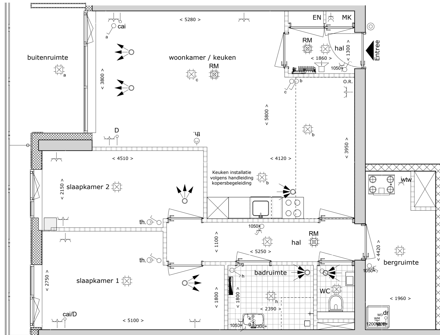
Bouwnummer A018 1 : 50
