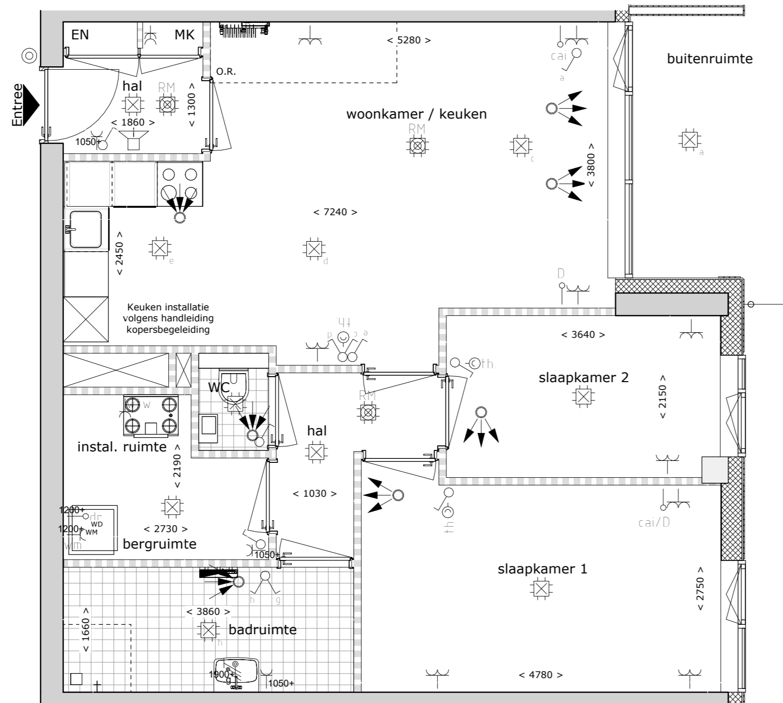
Bouwnummer A022 1 : 50
