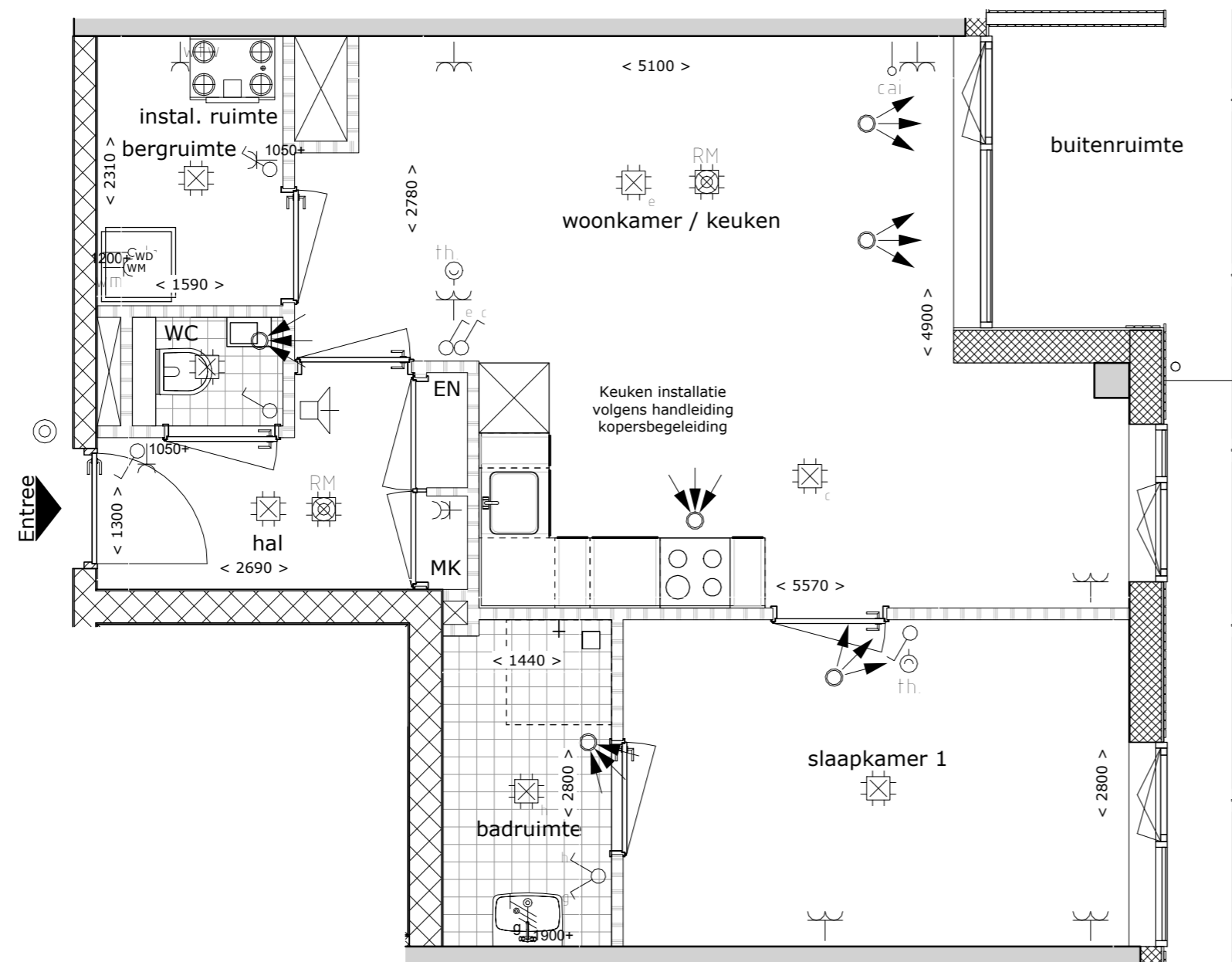
Bouwnummer A024 1 : 50
