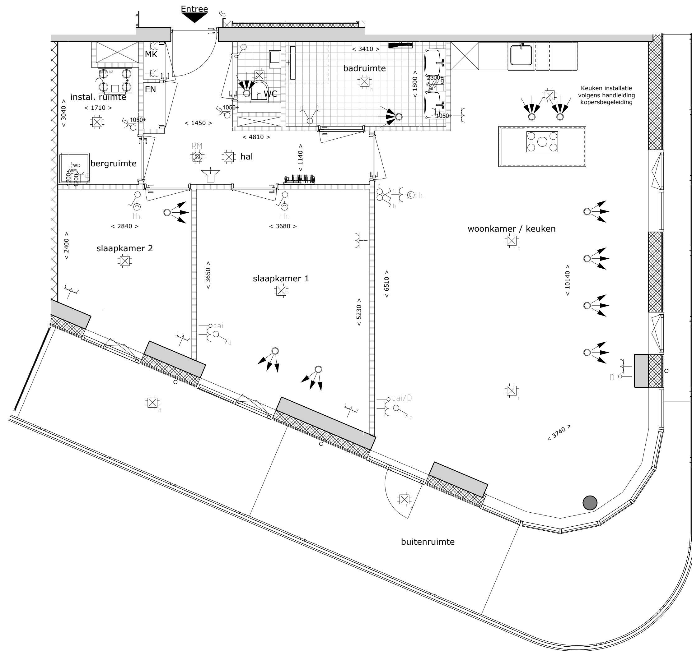
Bouwnummer A025 1 : 50
