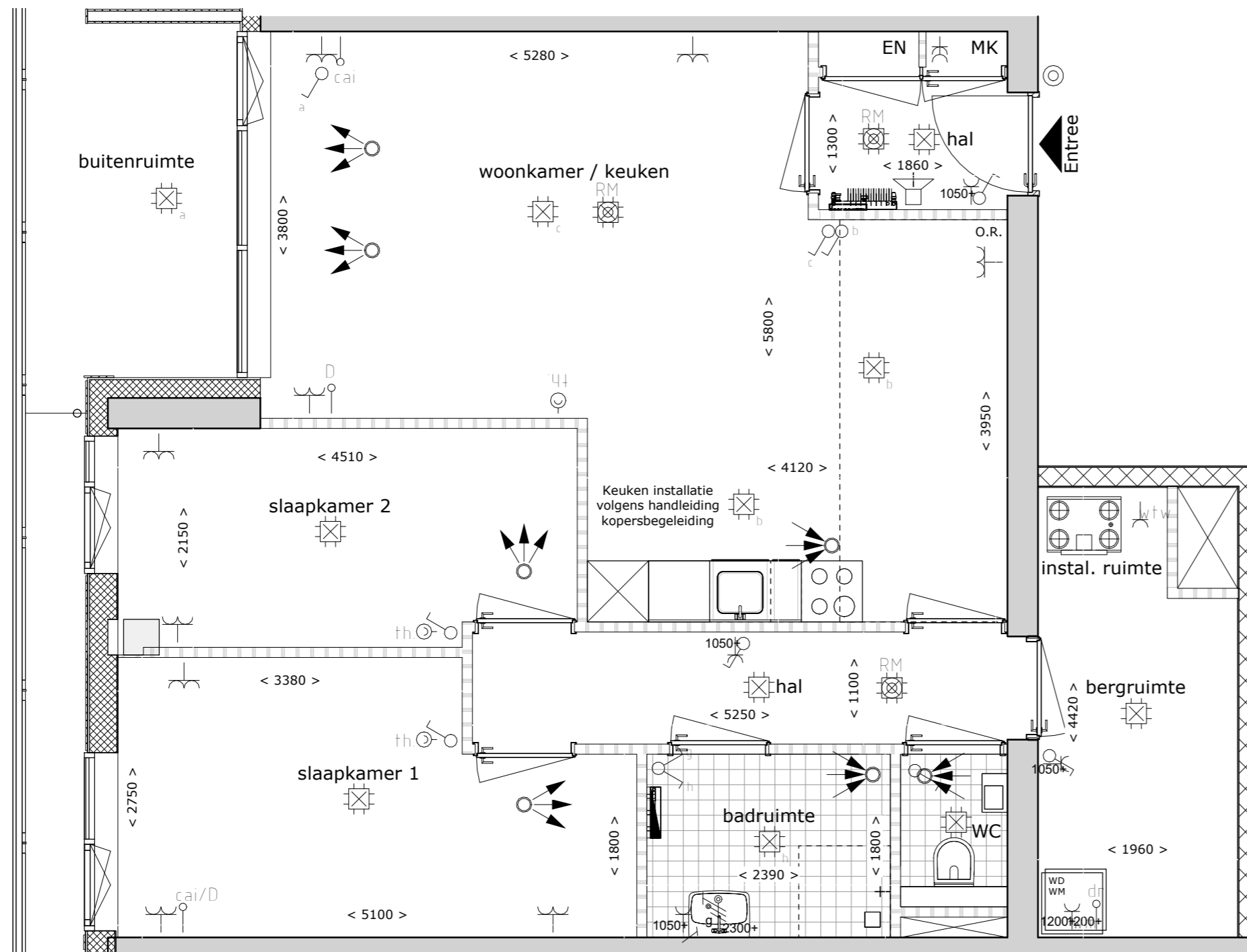
Bouwnummer A028 1 : 50
