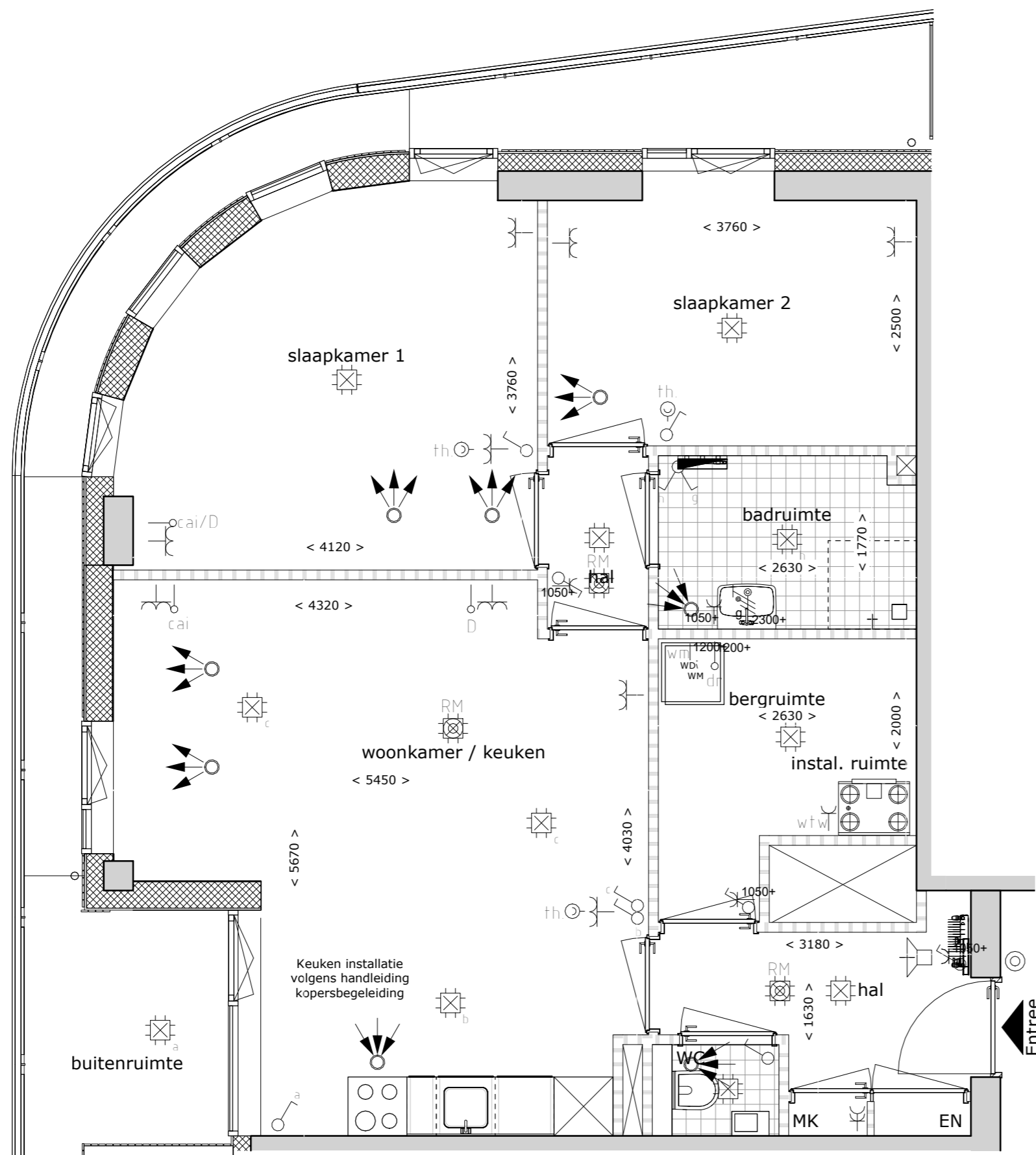
Bouwnummer A029 1 : 50
