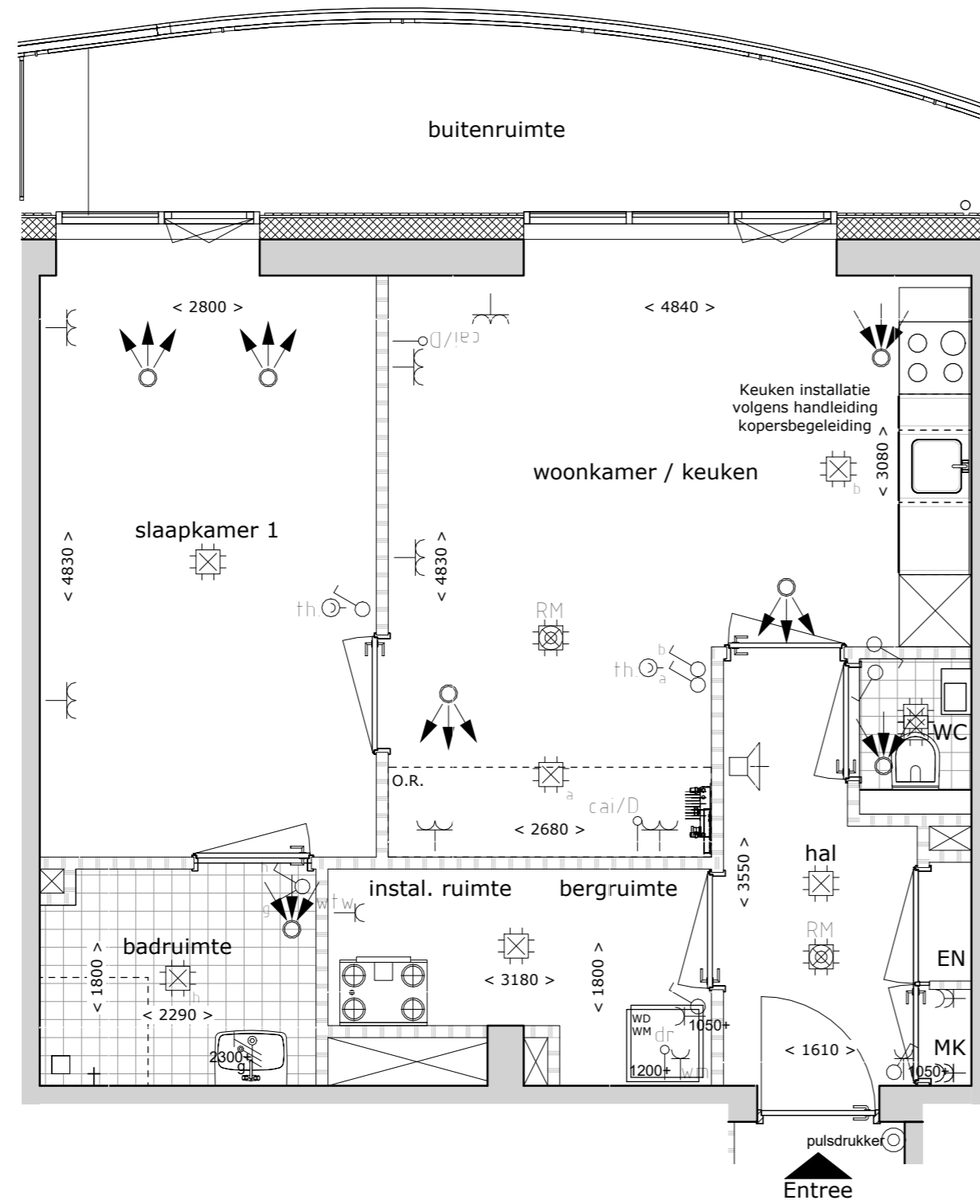
Bouwnummer A030 1 : 50
