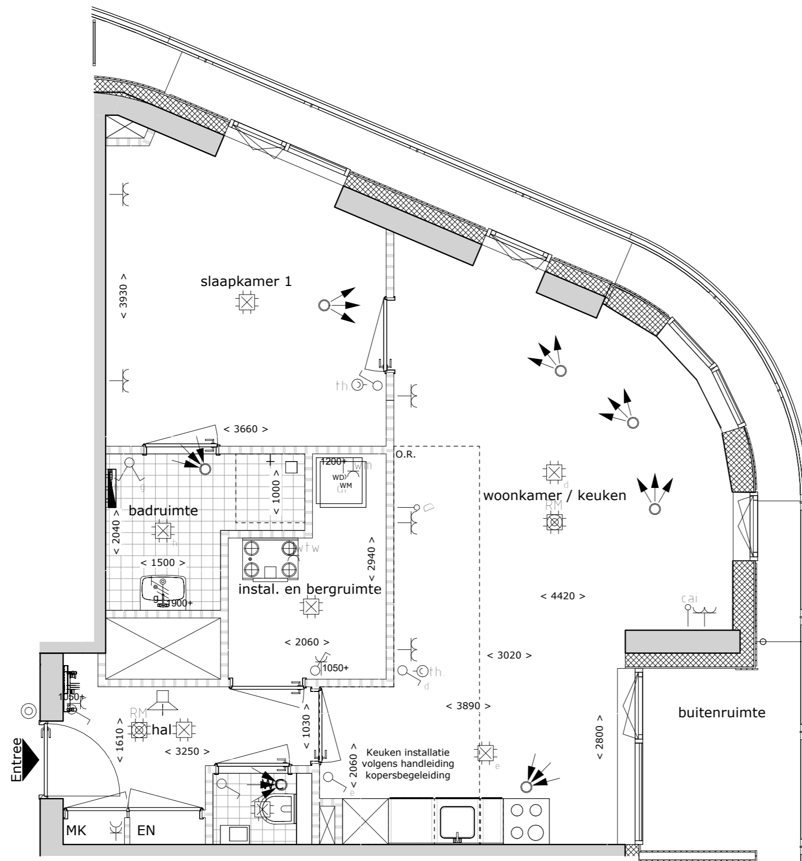
Bouwnummer A031 1 : 50
