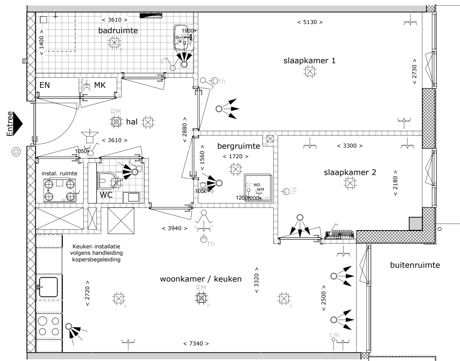
Bouwnummer A033 1 : 50
