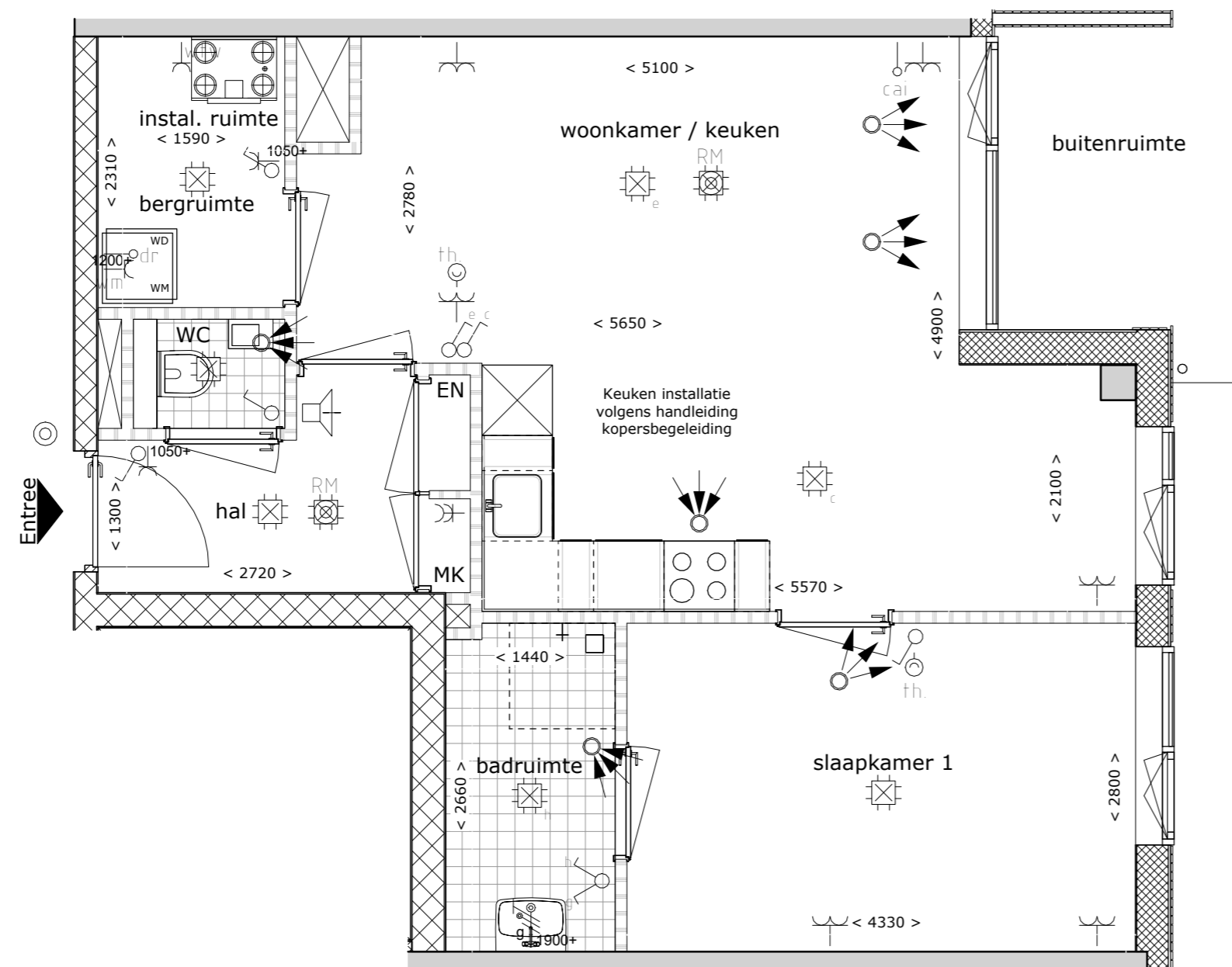
Bouwnummer A034 1 : 50
