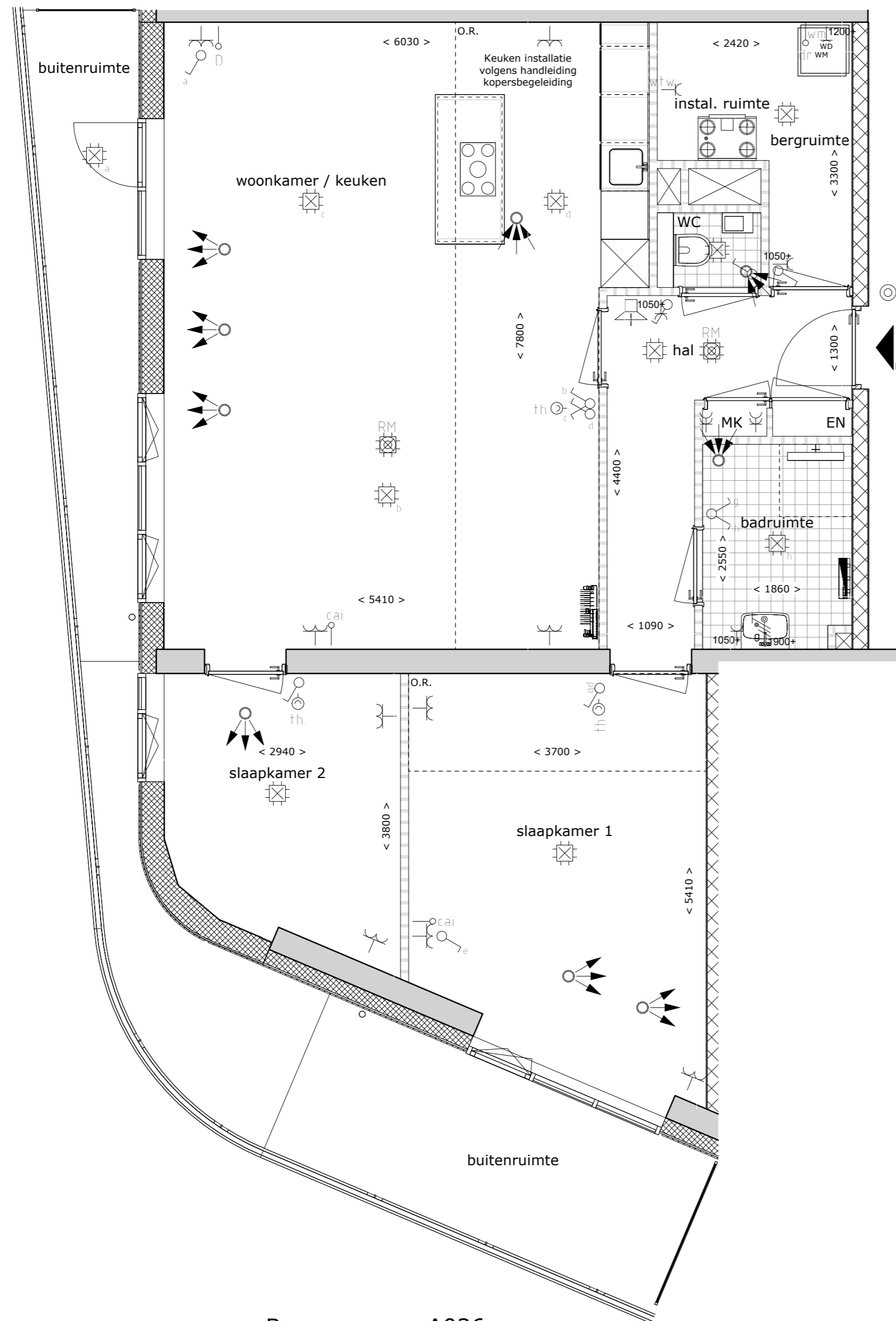
Bouwnummer A036 1 : 50
