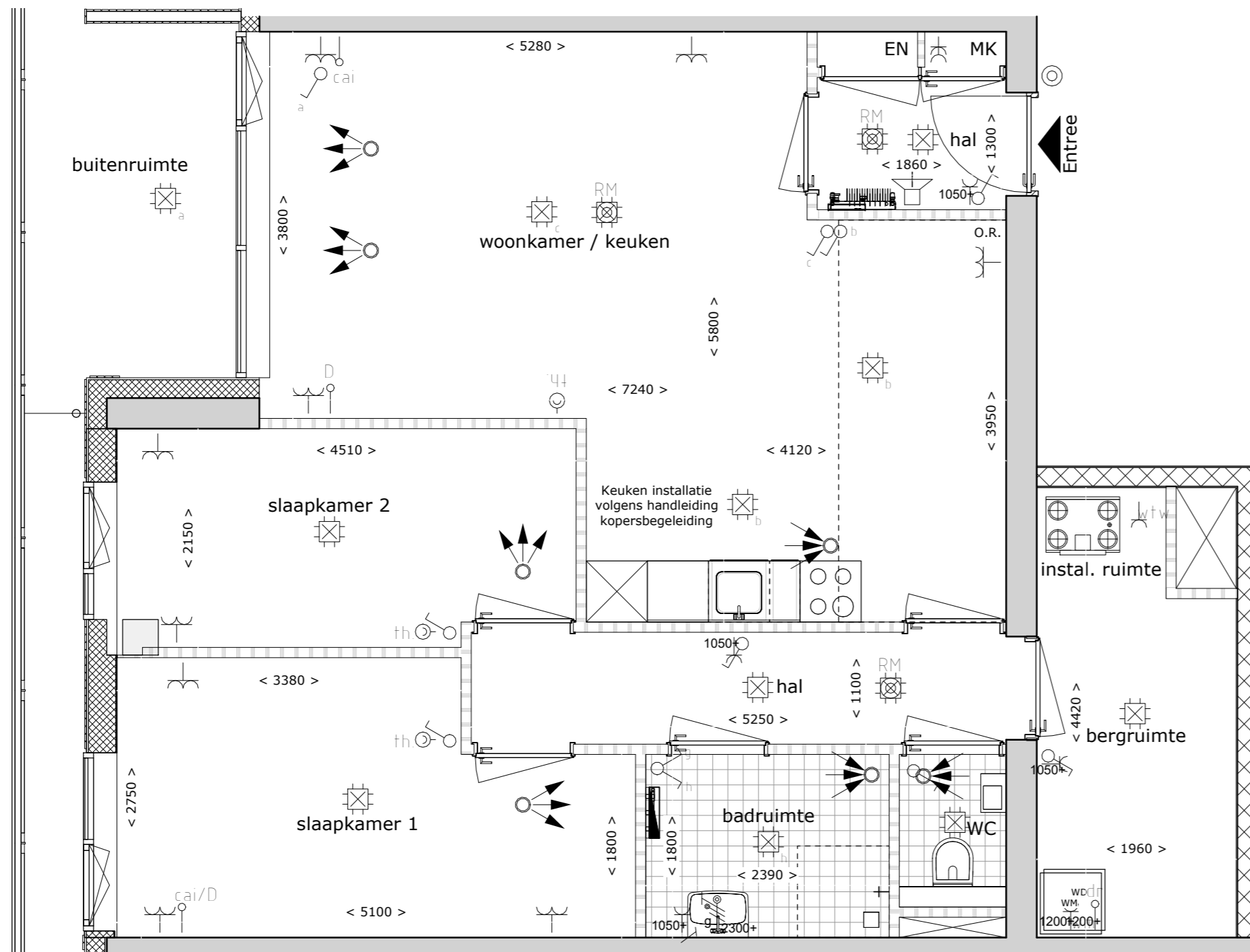
Bouwnummer A038 1 : 50
