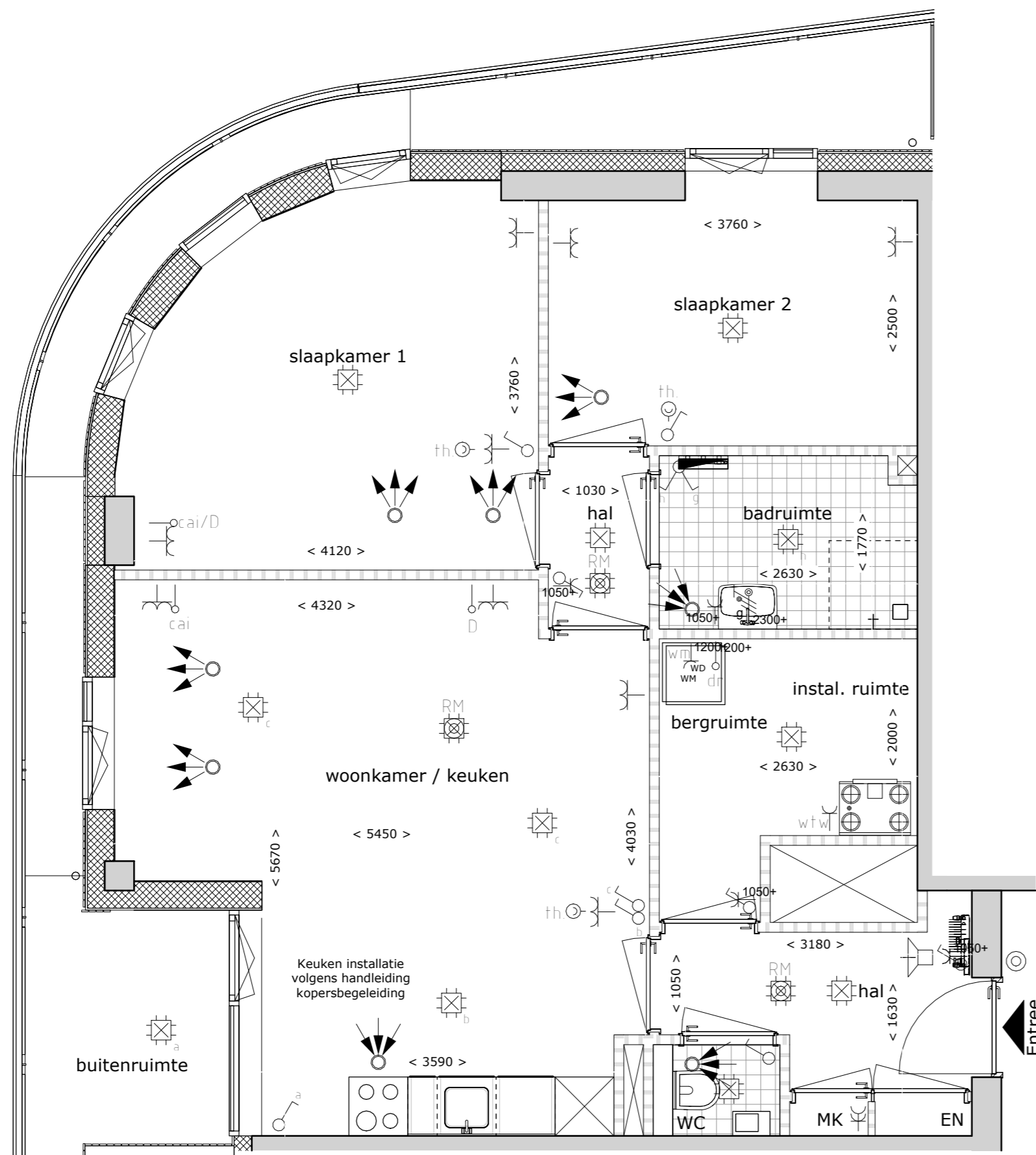
Bouwnummer A039 1 : 50
