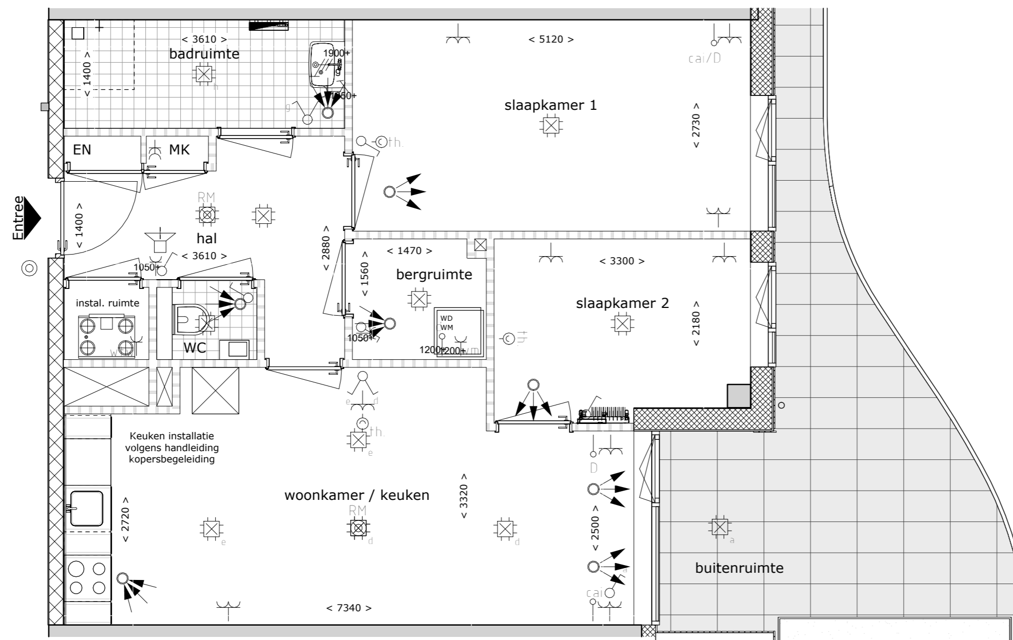
Bouwnummer A004 1 : 50
