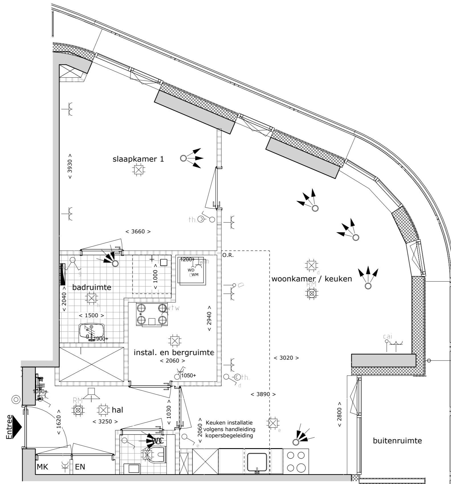
Bouwnummer A041 1 : 50
