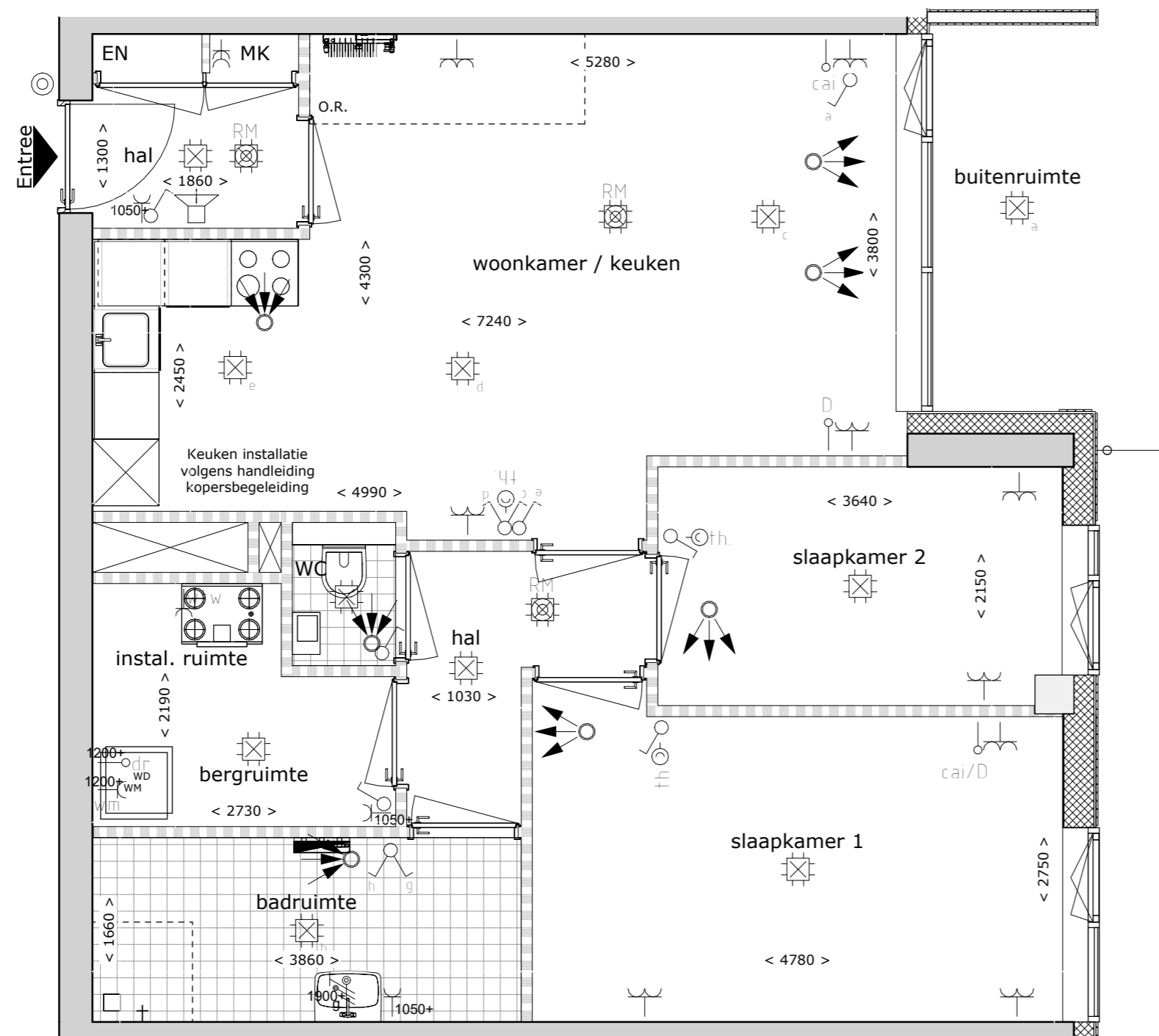
Bouwnummer A042 1 : 50
