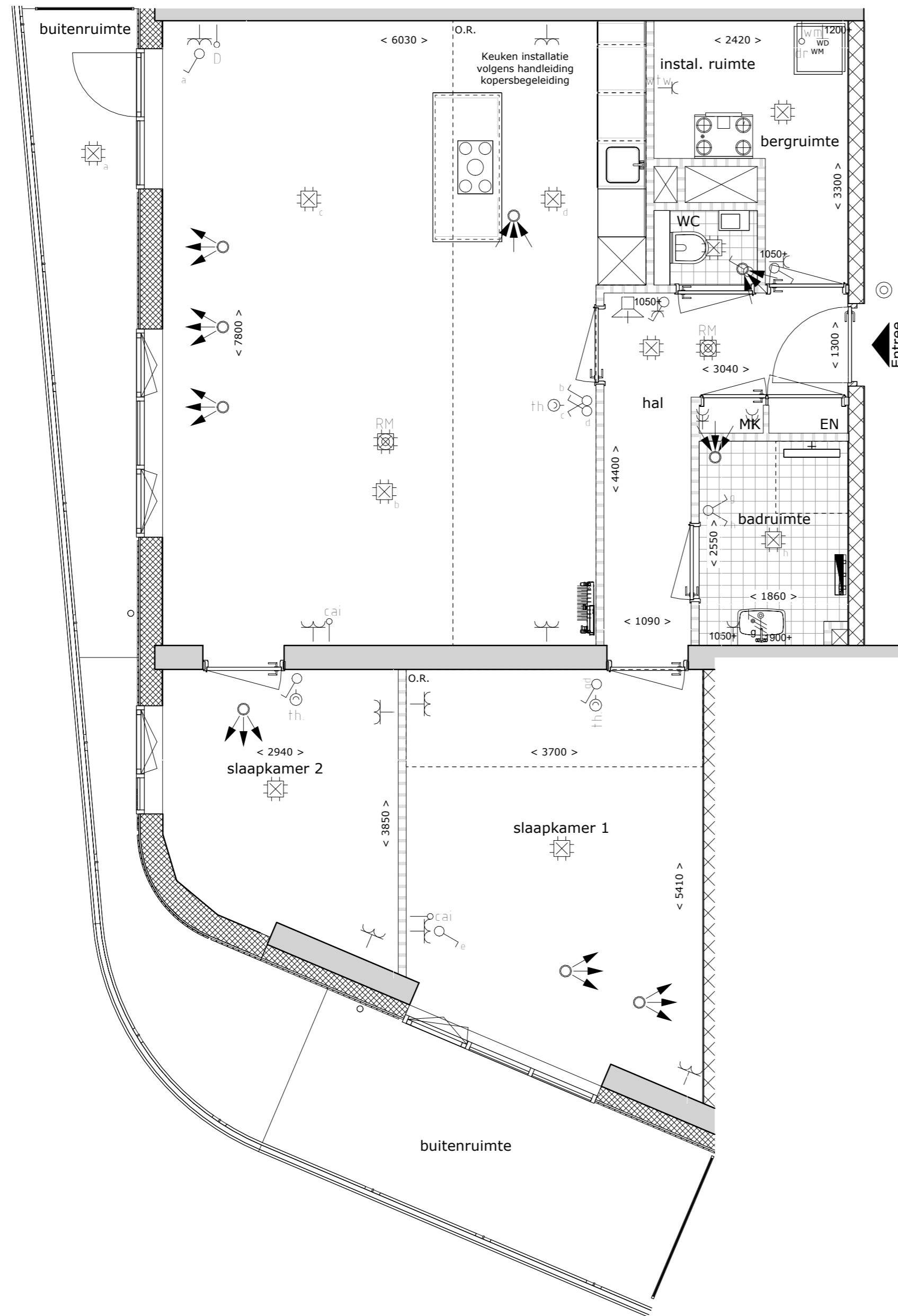
Bouwnummer A046 1 : 50
