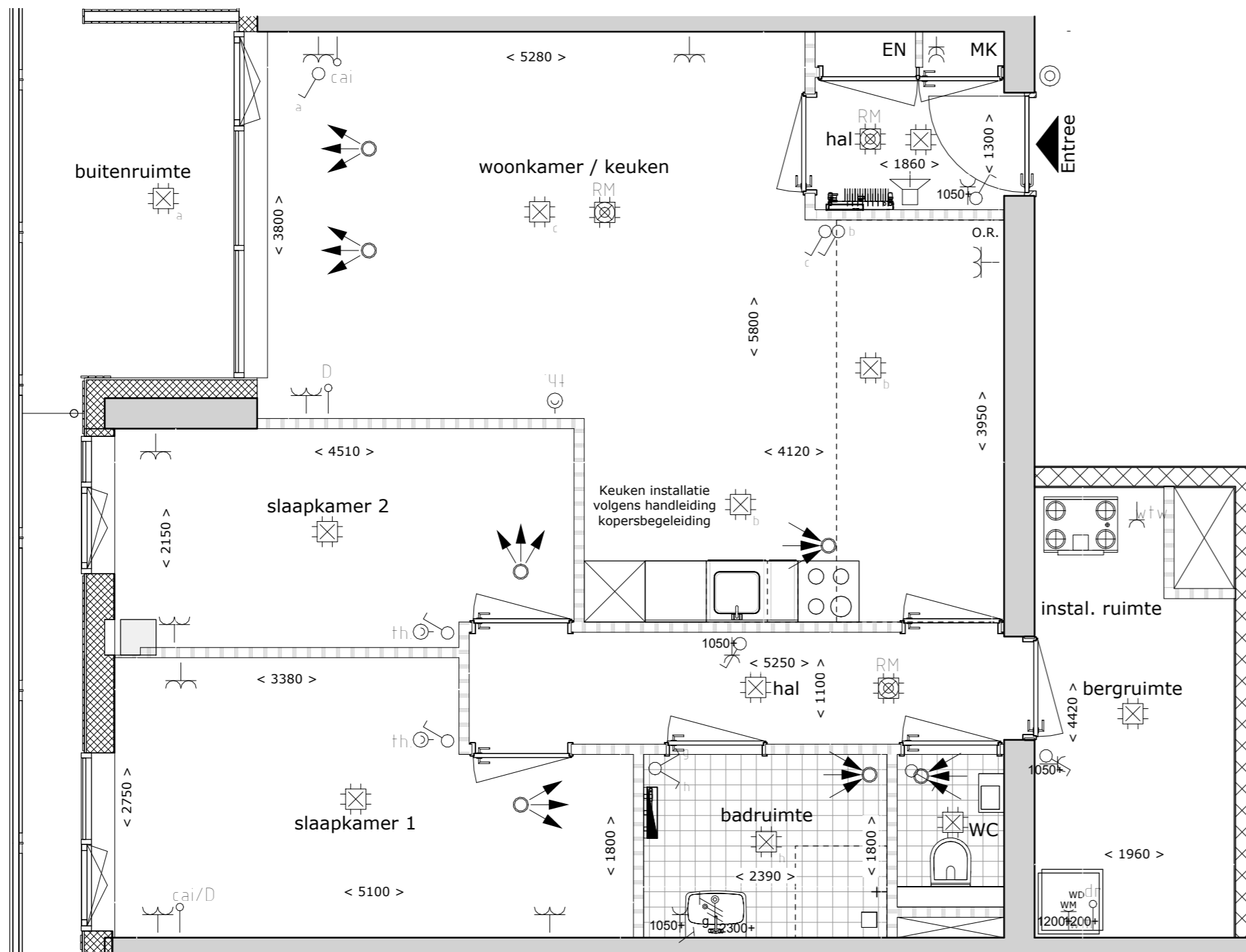
Bouwnummer A048 1 : 50
