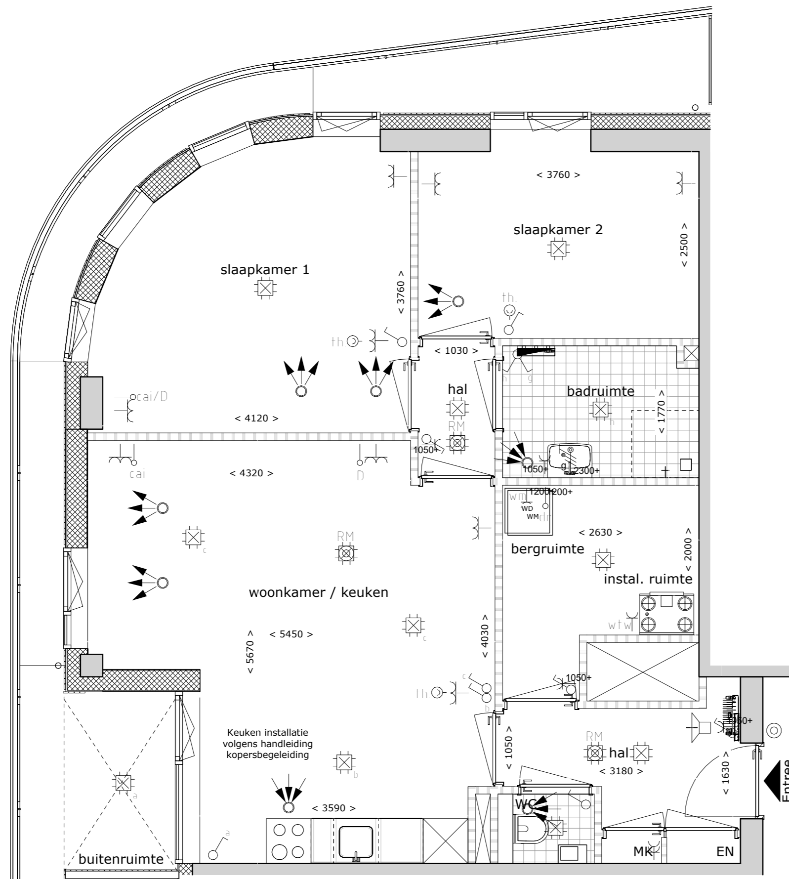
Bouwnummer A049 1 : 50
