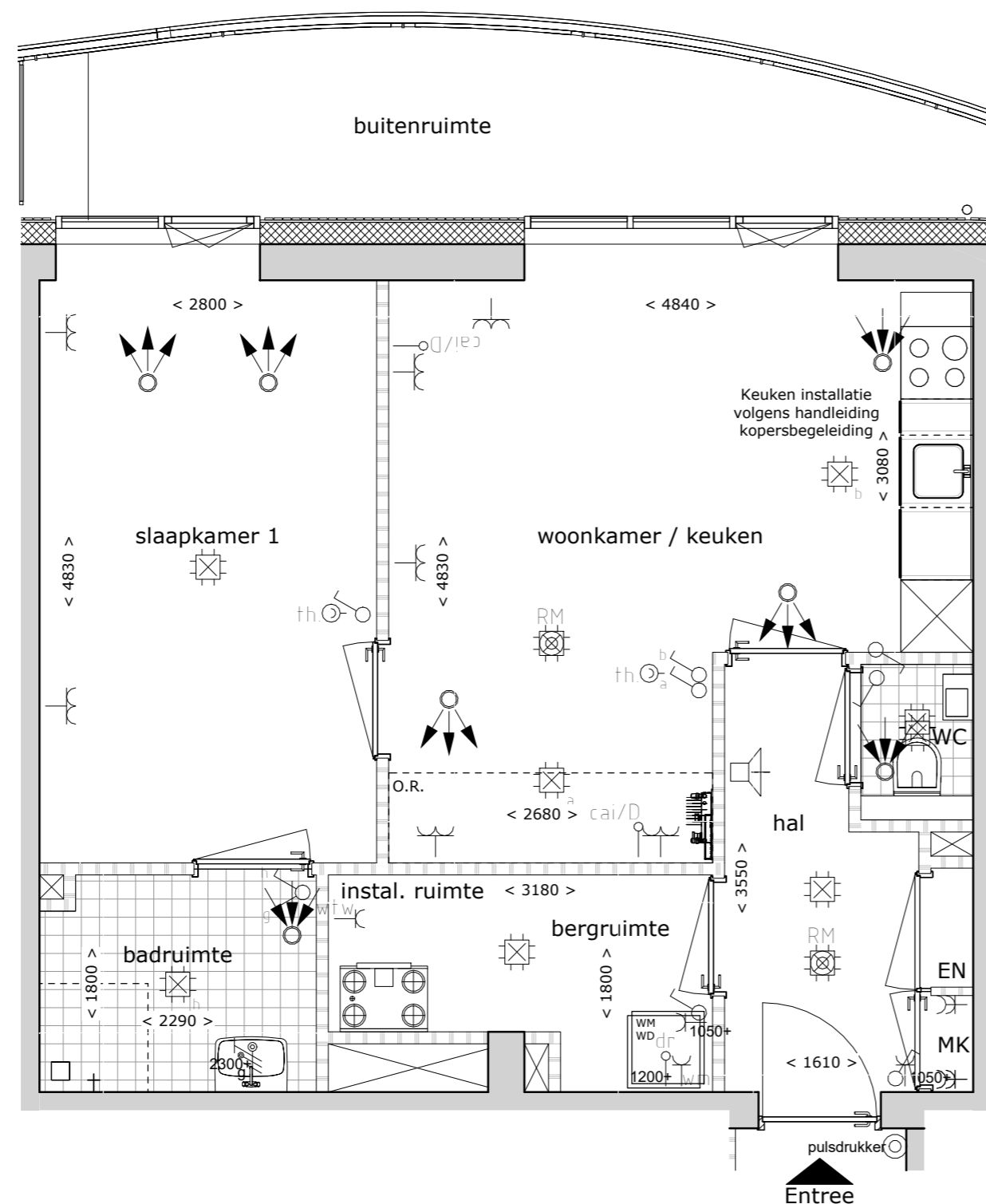
Bouwnummer A050 1 : 50
