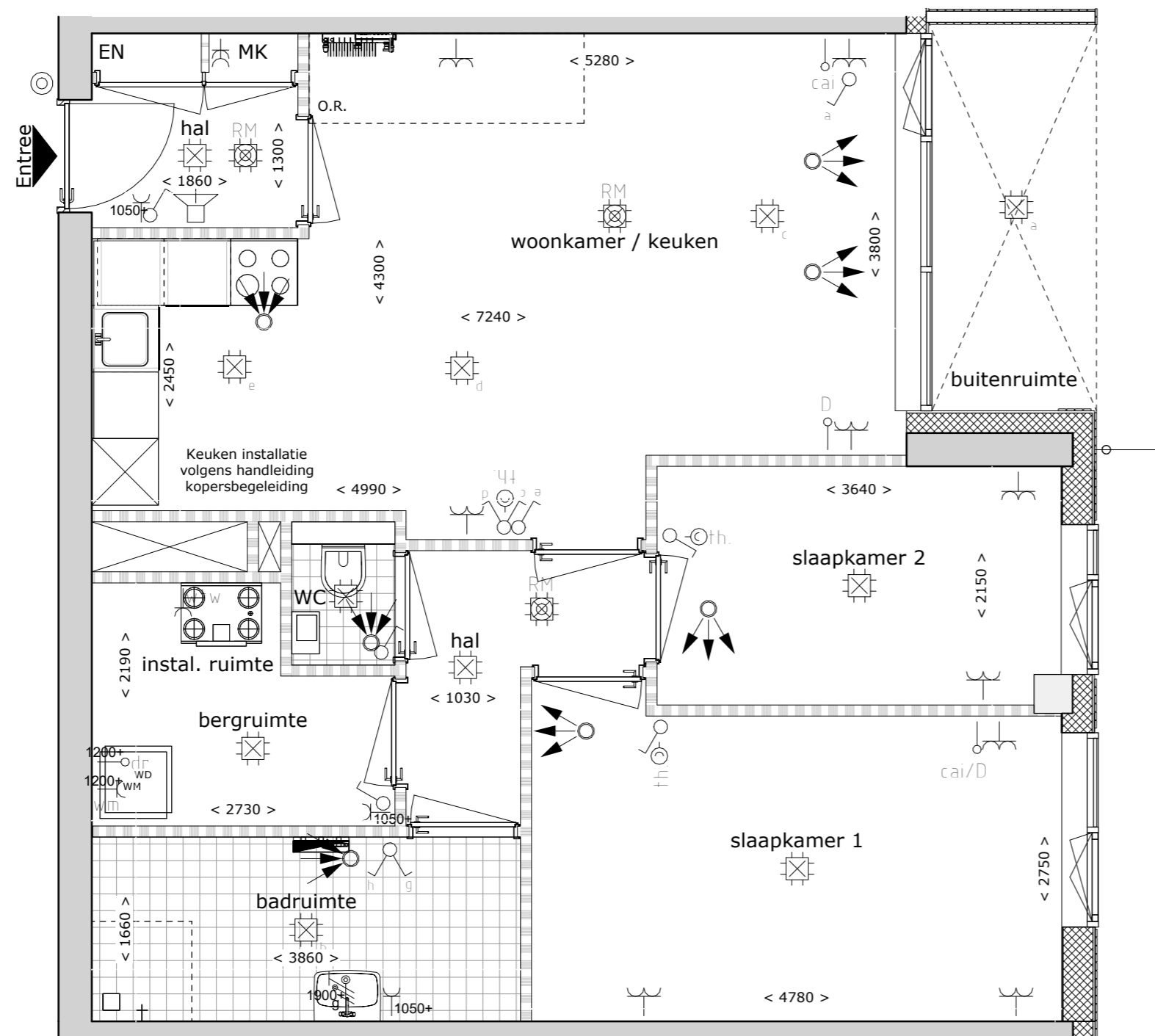
Bouwnummer A052 1 : 50
