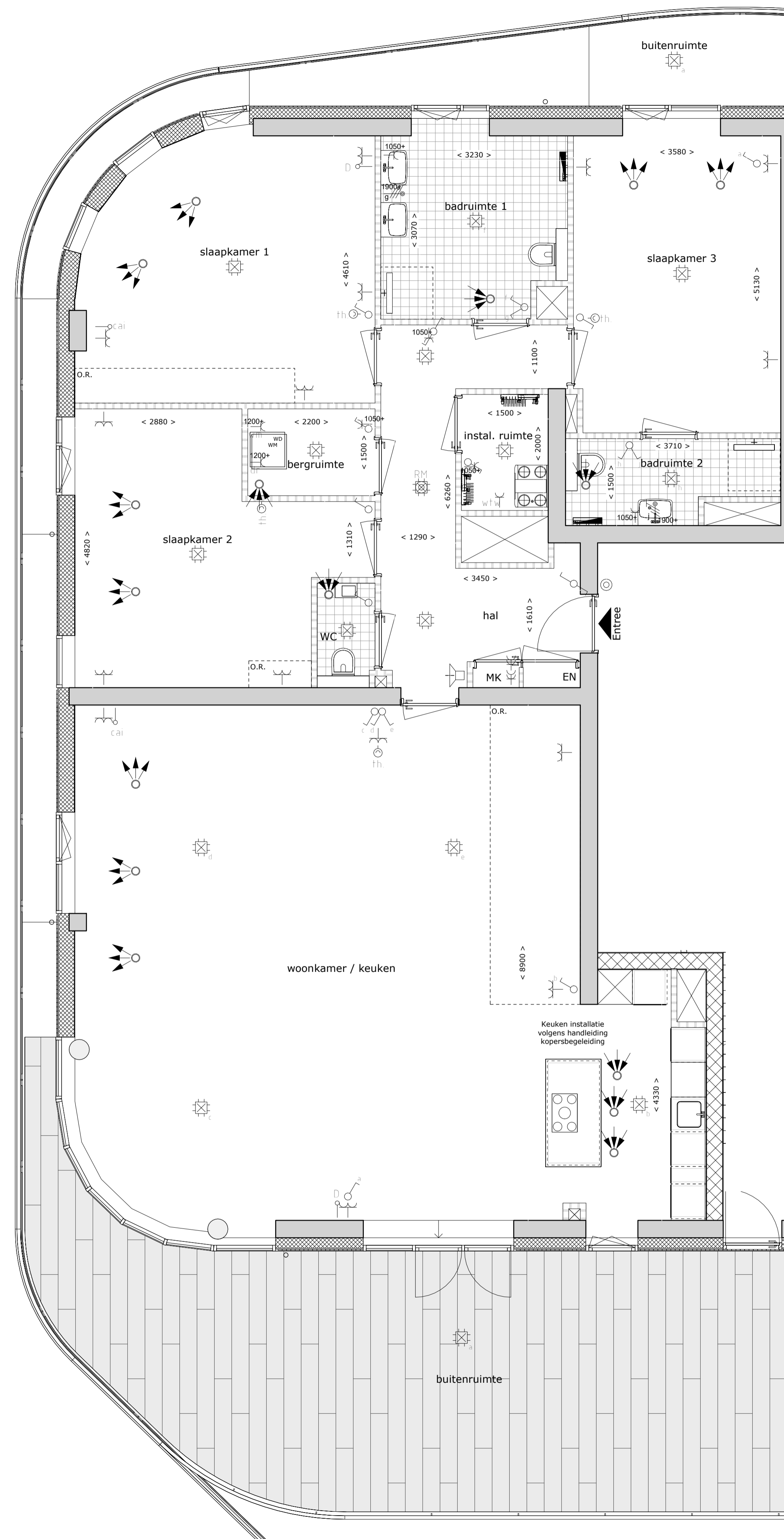
Bouwnummer A059 1 : 50
