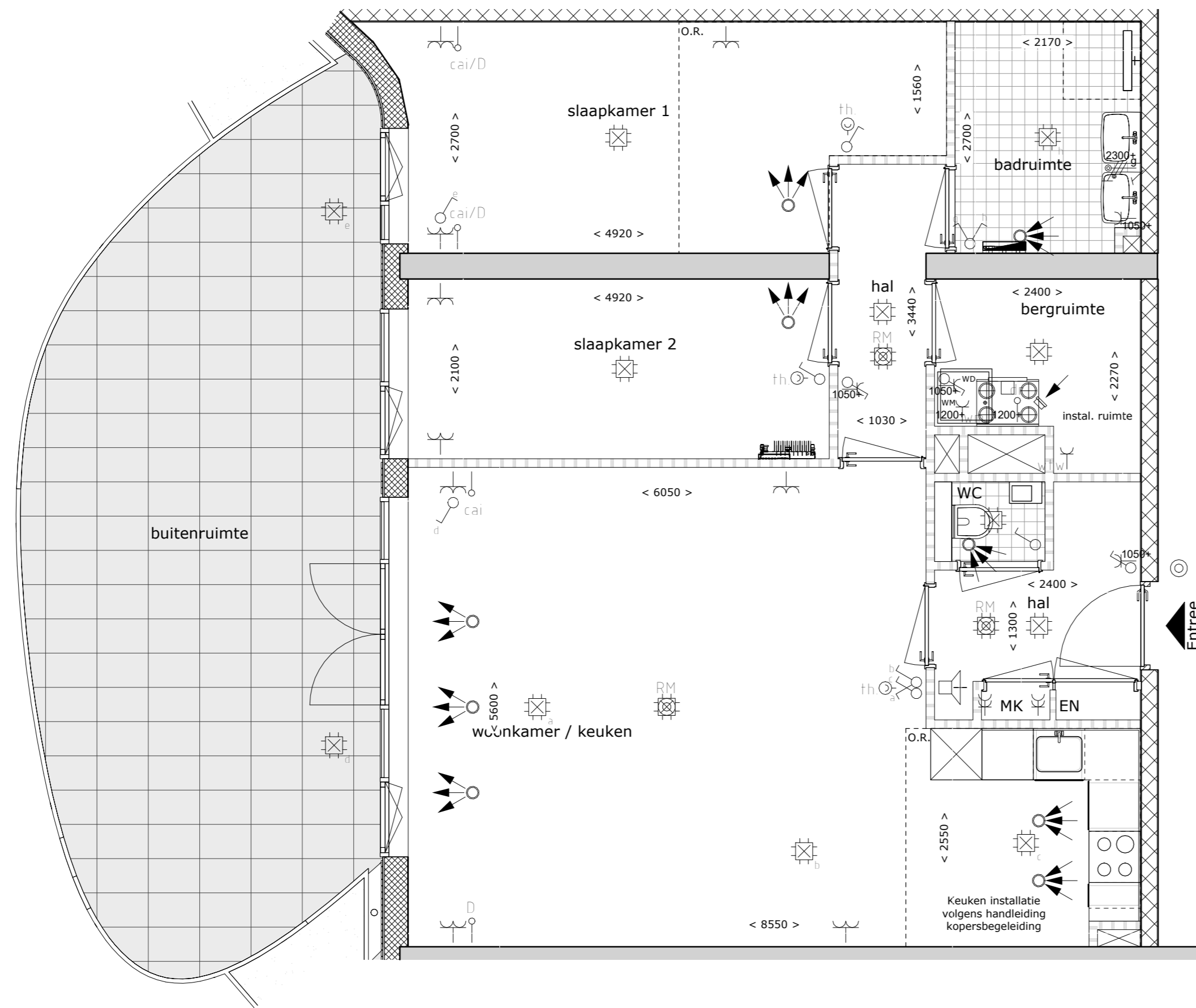
Bouwnummer A007 1 : 50
