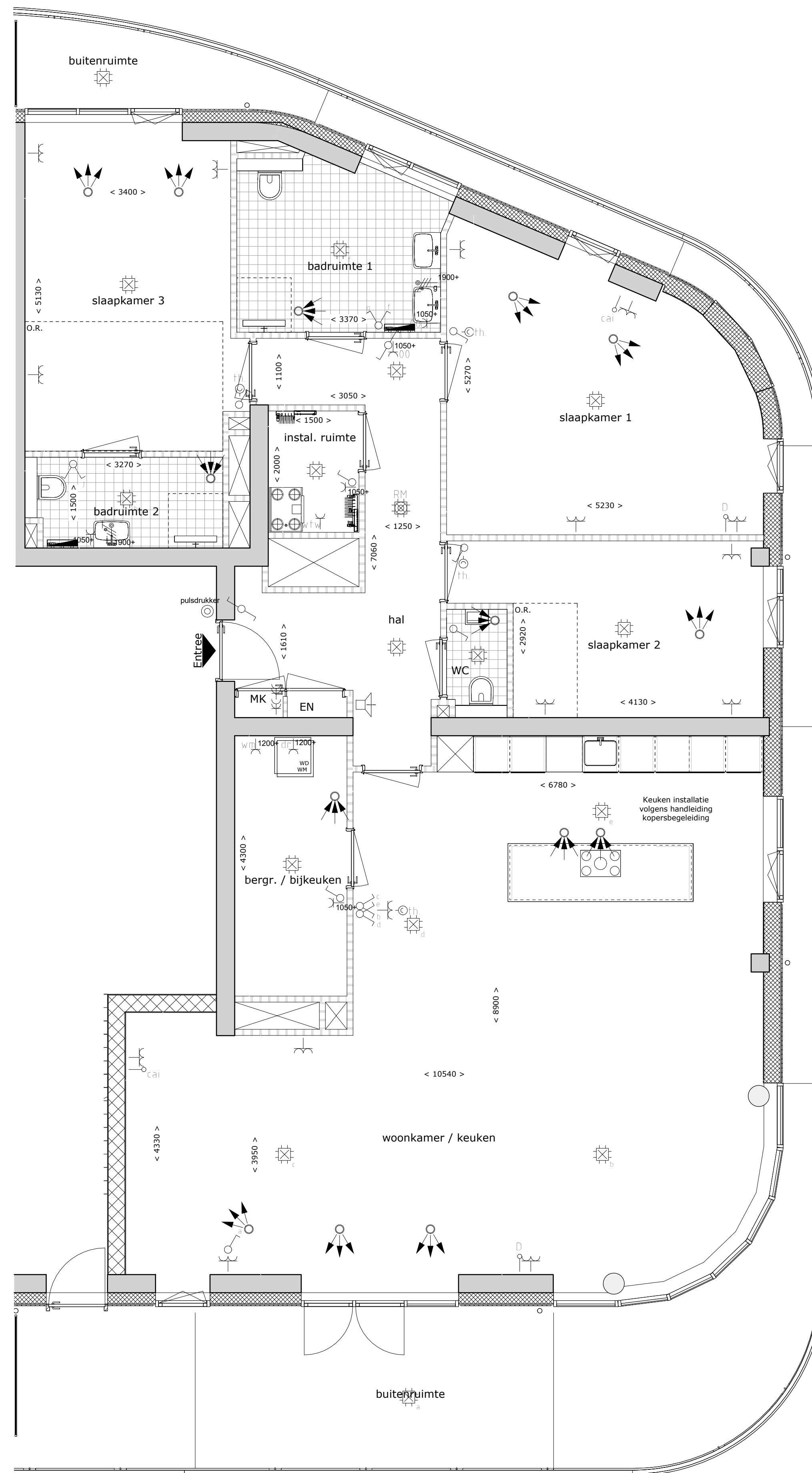
Bouwnummer A062 1 : 50
