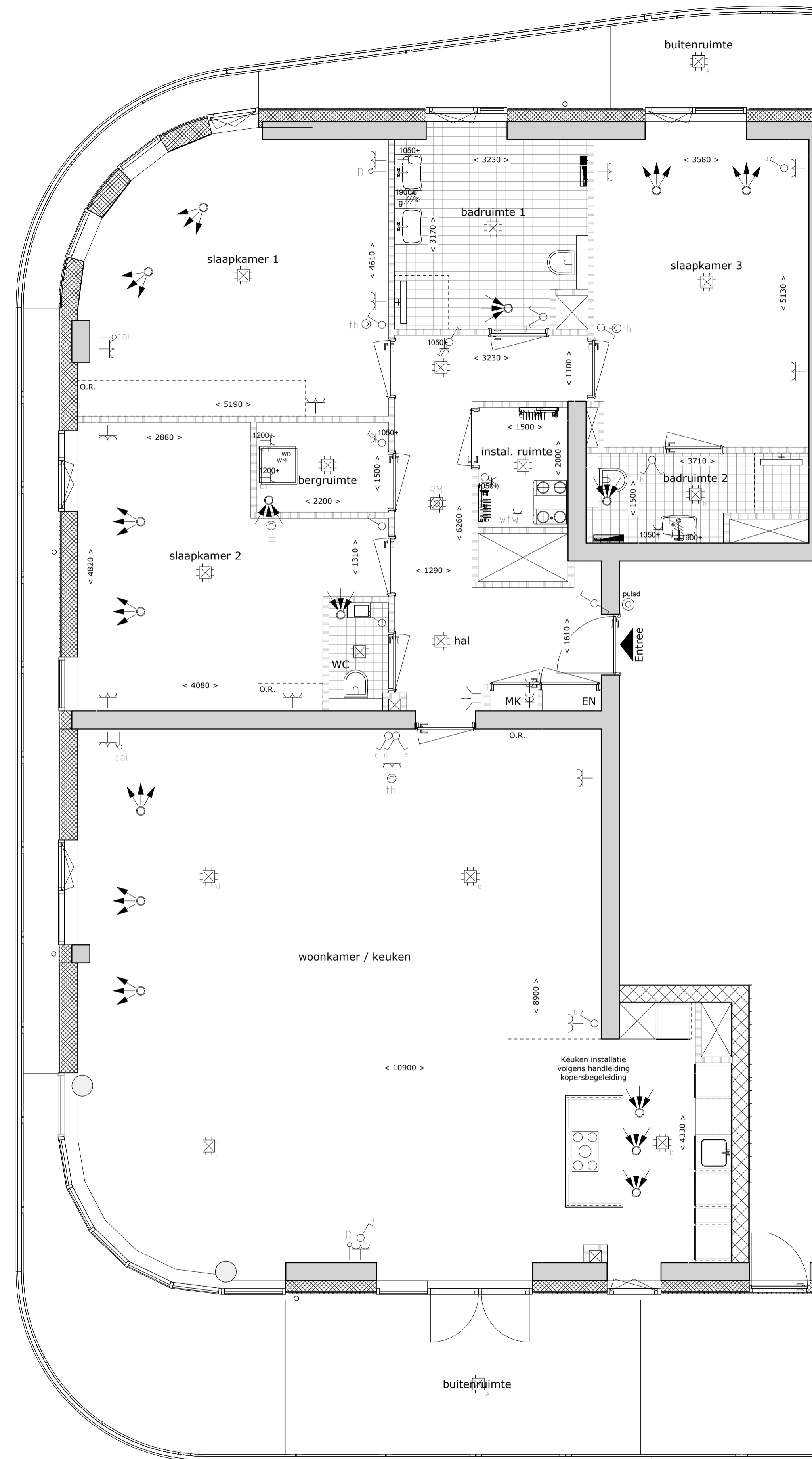
Bouwnummer A063 1 : 50
