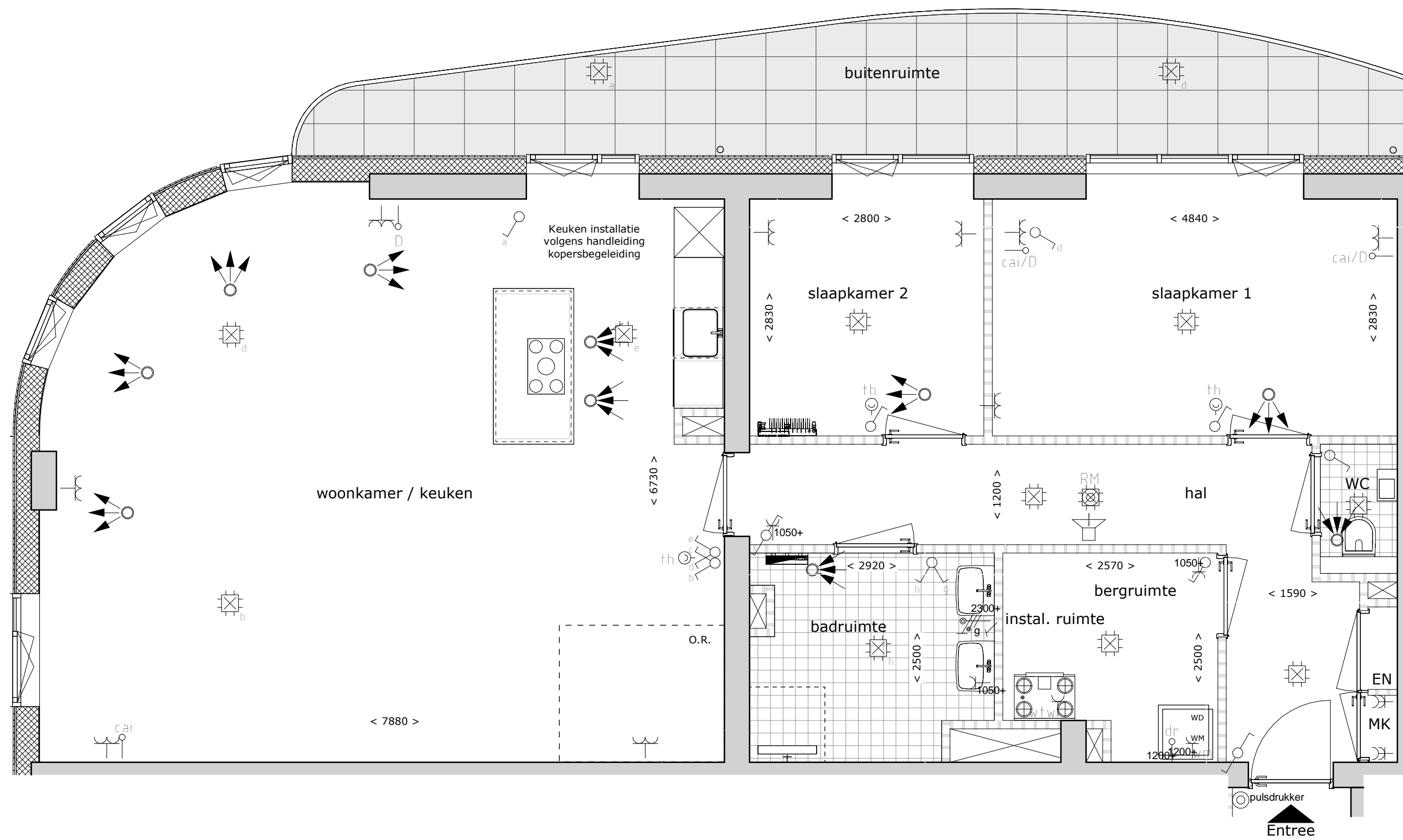
Bouwnummer A001 1 : 50
